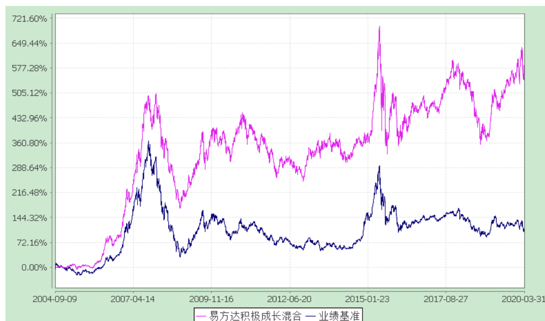
易方达积极成长证券投资基金 累计净值增长率与业绩比较基准收益率的历史走势对比图 (2004 年 9 月 9 日至 2020 年 3 月 31 日)
